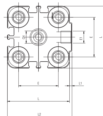
Ø 32-40-50-63-80-100
