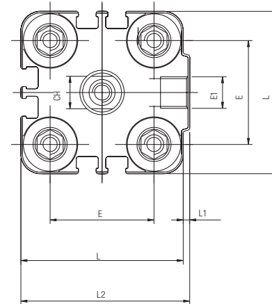
Ø 32-40-50-63-80-100
